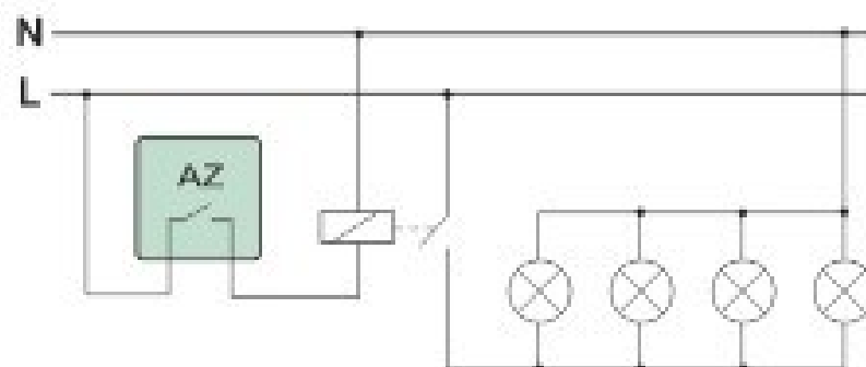
Układ sterowania słycznkiem złączającym odbiorniki o łącznym poborze prądu przewyższającym dopuszczalne obciążenie styku automatu zmierzchowego
